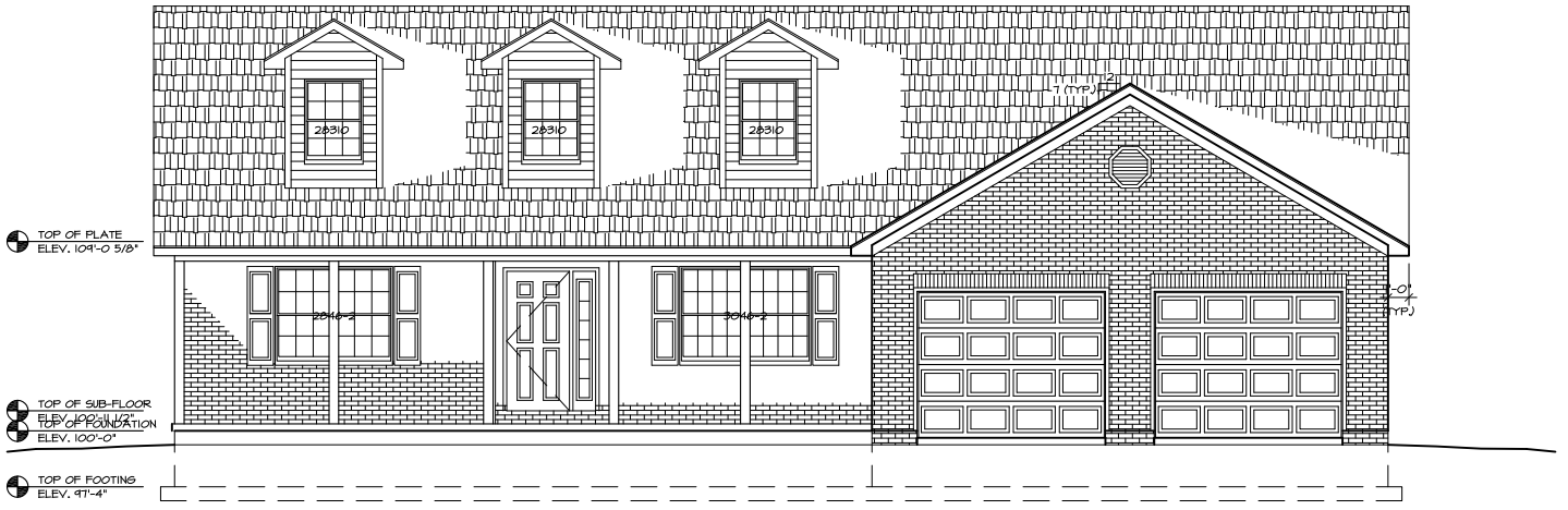
1 FRONT ELEVATION A-1 SCALE: 1/4"=1'-0"
